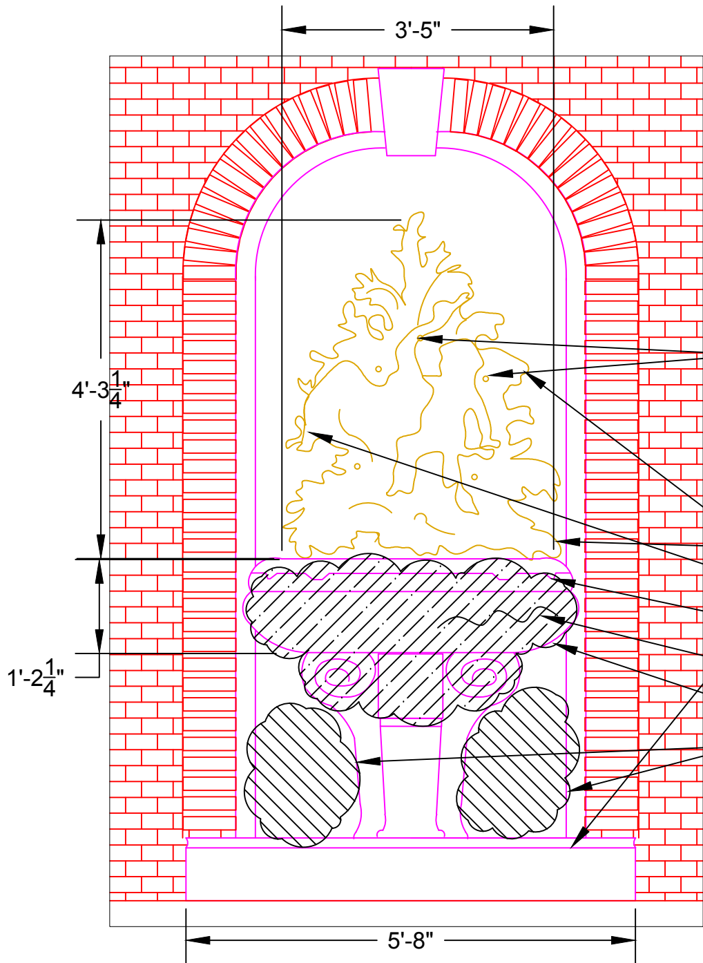
ELEVATION
